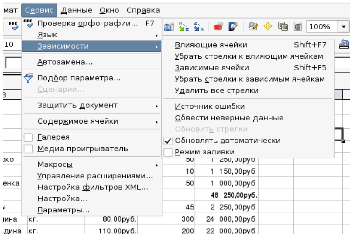
Рисунок 29 – Зависимости формул
